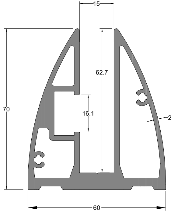
Cam Kanallı Küpeşte Profili GLAZING HANDRAIL PROFILE
